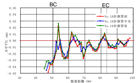
図-3 推進管の水平偏差（+：左向き）
