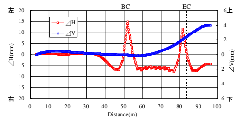
図-4 推進管偏差
