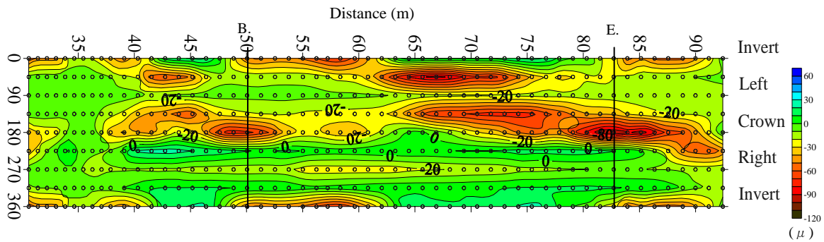
図-2 管軸方向内周面ひずみの時系列変化（計測管 No. 18, A 断面）（-：圧縮，○：計測位置）
