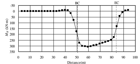
図-5 水平曲げモーメント
