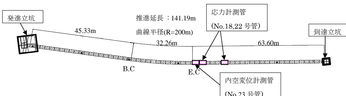
図-1 現場平面図（到達時）
