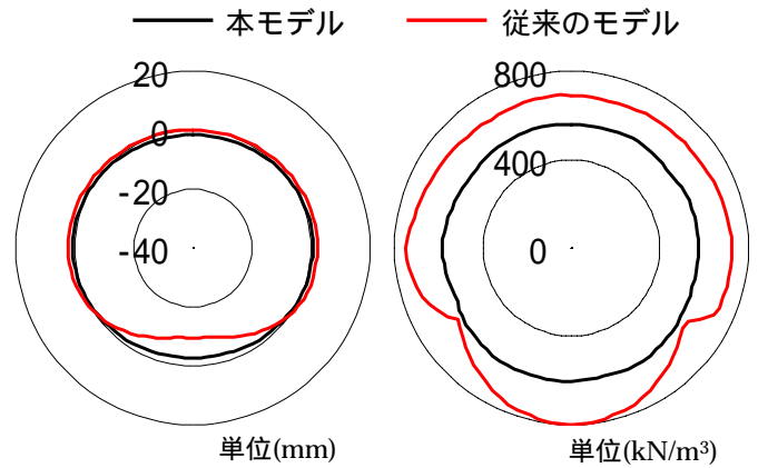
図8 変位分布図 図9 作用土水圧分布図
