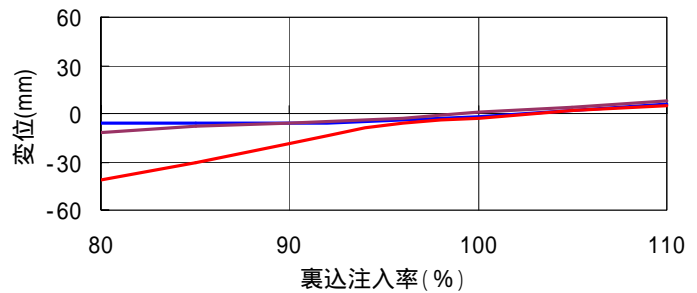
図6 変位 - 裏込注入率
