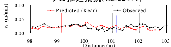
図11 掘進速度(Case2071)
