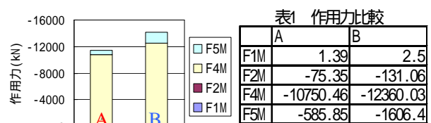
図12 作用力比較(Case2071)
