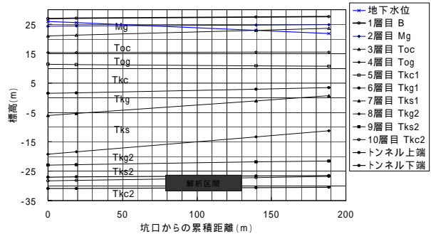
図 4 地質縦断図
